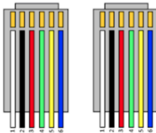
RJ12 Pegasus Controller RJ12 MSM Motor
